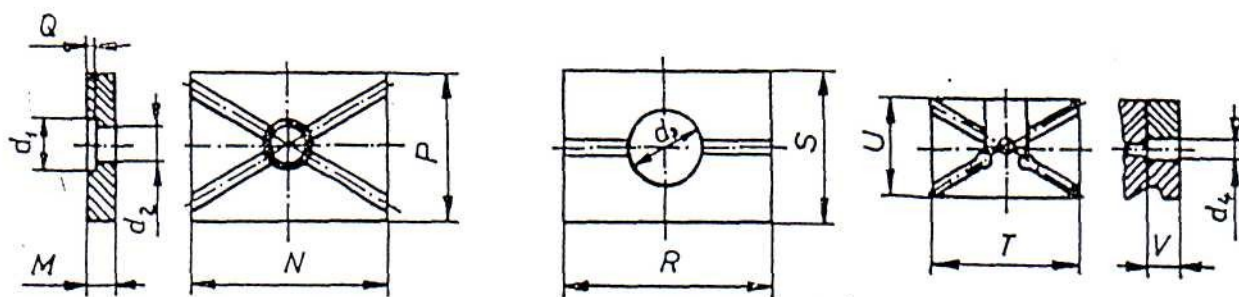
I. Felfogólap ①
